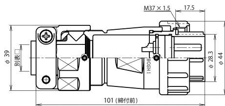
NJW-32 ■ -PM □
