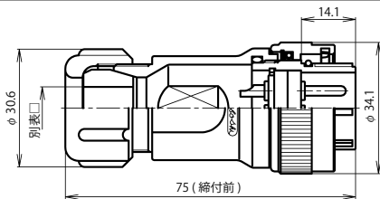
NRW-24 ■ -PM □
