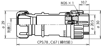
NJW-24 ■ -PM □
