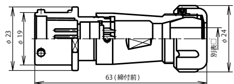
NAW-16 ■ -AdM □
