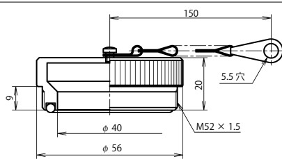
プラグキャップ：NWPC-44-PCa
