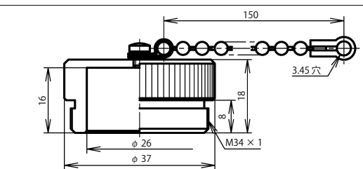
プラグキャップ：NWPC-30-PCa
