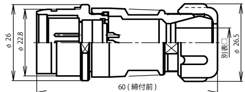
NRW-20 ■ -AdM □
