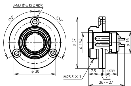
NWPC-16 ■ -R-CH
