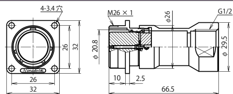
NJW-24 ■ -GAd(F)F1/2 (注)
