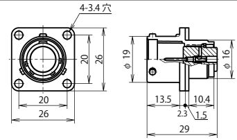
NAW-16 ■ -RM
