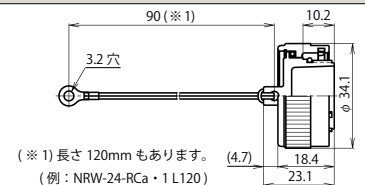
レセプタクル防水キャップ: NRW-24-RCa・1
