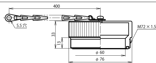
プラグキャップ: 64EUMW-PCa
