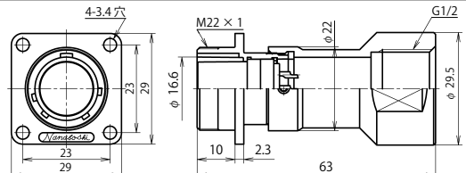
NJW-20 ■ -GAd(F)F1/2 (注)
