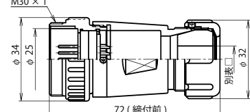
NJW-28 ■ -AdM □
