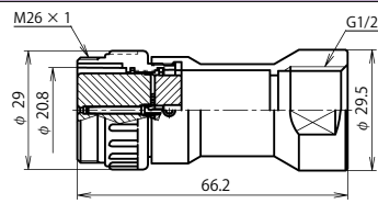
NJW-24 ■ -GAdF1/2 (注)
