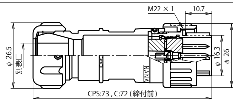
NJW-20 ■ -PM □
