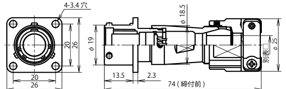
NAW-16 ■ -Ad(F)FK □
