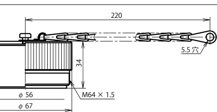
プラグキャップ：NWPC-60-PCa
