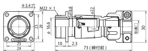
NJW-20 ■ -Ad(F)FK □
