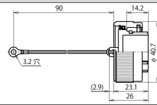
レセプタクル防水キャップ：NRW-28-RCa・1
