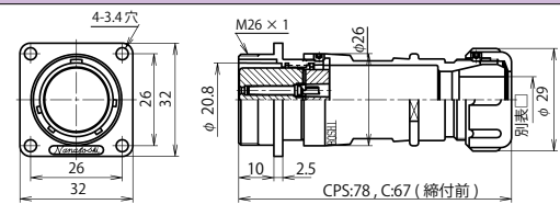
NJW-24 ■ -Ad(F)F □
