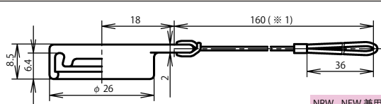
レセプタクルゴムキャップ：NRW-20-RCa・2
