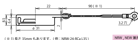
レセプタクルゴムキャップ：NRW-24-RCa
