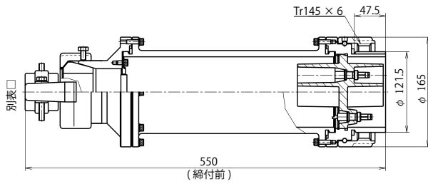
プラグ ソケット(メス)コネクタ NHVC-1204-6V-PF
