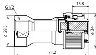
NAW-24 ■ -GPF1/2 (注)
