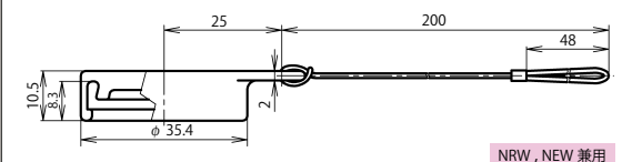
アダプタゴムキャップ：NRW-28-AdCa
