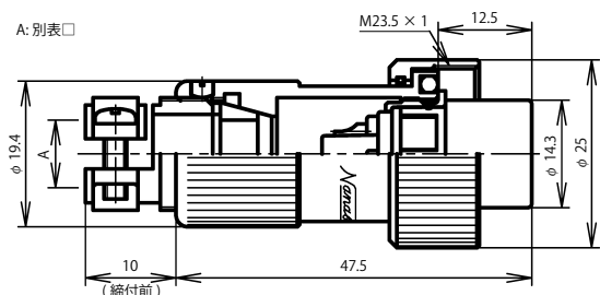
NWPC-16 ■ -P □ -CH
