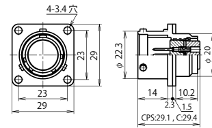
NAW-20 ■ -RM
