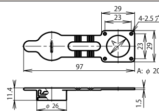
レセプタクルゴムキャップ：NRW-20-RCa・2
