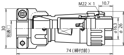
NJW-20 ■ -PFK □
