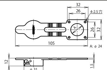
レセプタクルゴムキャップ: NRW-24-RCa・2
