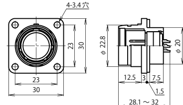
NRW-20 ■ -RM
