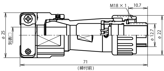
NJW-16 ■ -PFK □
