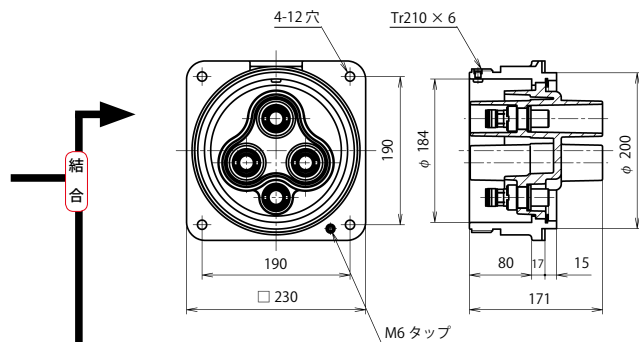
ソケット(メス)コンタクト
