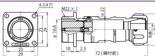
NJW-20 ■ -Ad(F) □
