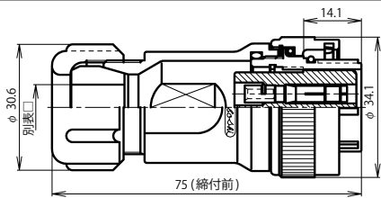
NRW-24 ■ -PF □
