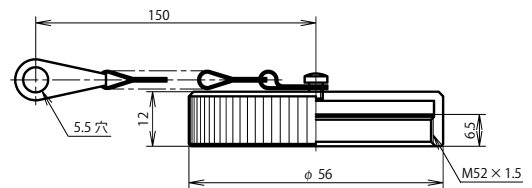
アダプタキャップ：NWPC-44-AdCa
