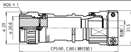
NJW-24 ■ -AdFK □
