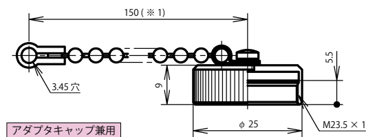
レセプタクルキャップ：NWPC-16-RCa
