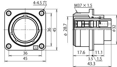
NJW-32 ■ -RF
