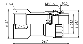
NJW-28 ■ -GPF3/4 (注)
