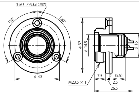
NWPC-16 ■ -RF-CH
