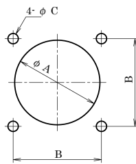
角フランジ付きアダプタ（4点穴）
