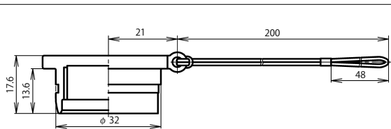
プラグ防水キャップ：NRW-28-PCa・1
