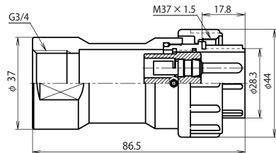
NJW-32 ■ -GPM3/4 (注)
