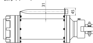
オプション部品取り付けイメージ
