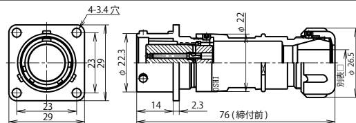
NAW-20 ■ -Ad(F)F □
