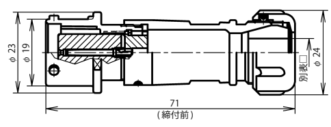
NAW-16 ■ -AdF □
