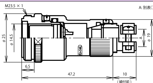
NWPC-16 ■ -AdF □ -CH
