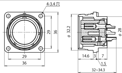
NEW-28 ■ -RF
