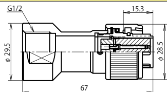
NAW-20 ■ -GPF1/2 (注)
