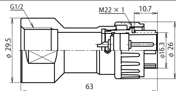
NJW-20 ■ -GPM1/2 (注)
