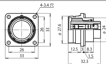
NRW-24 ■ -RF
