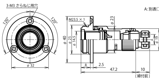
NWPC-16 ■ -AdF(F) □ -CH
