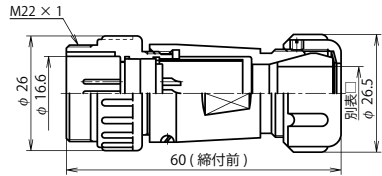
NJW-20 ■ -AdM □
