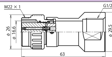
NJW-20 ■ -GAdF1/2 (注)
