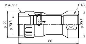
NJW-24 ■ -GAdF1/2 (注)
