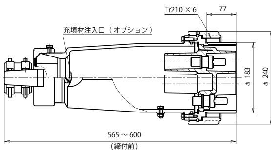
ピン(オス)コンタクト
