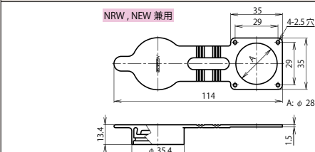
レセプタクルゴムキャップ：NRW-28-RCa・2
