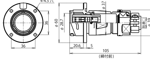
BWC-32 ■ -Ad(F)F □
