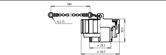
アダプタキャップ：BWC-32-AdCa
