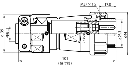
NJW-32 ■ -PM □
