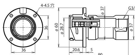
BWC-32 ■ -GAd(F)F3/4 (注)
