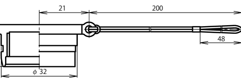
プラグ防水キャップ：NRW-28-PCa・1
