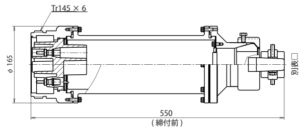
アダプタ ピン(オス)コネクタ NHVC-1204-6V-AdM
