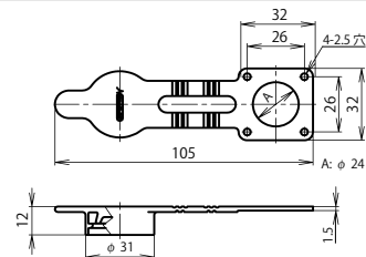
レセプタクルゴムキャップ: NRW-24-RCa・2
