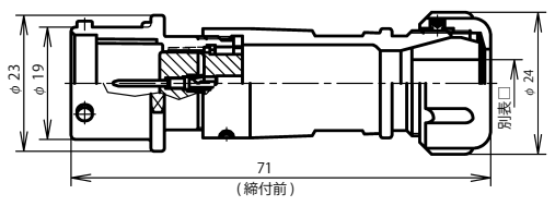
NAW-16 ■ -AdM □
