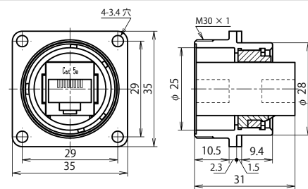
ENJW-28SC5E-R
