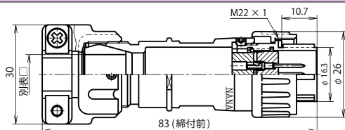
NJW-20 ■ -PMK □
