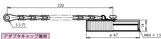
レセプタクルキャップ：NWPC-60-RCa
