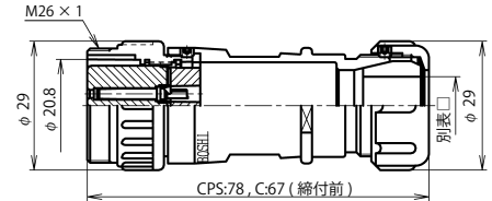
NJW-24 ■ -AdF □
