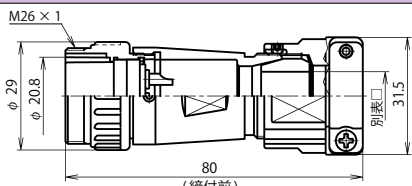
NJW-24 ■ -AdFK □
