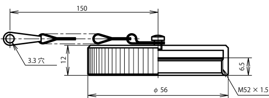
レセプタクルキャップ：NWPC-44-RCa
