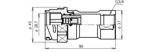
BWC-32 ■ -GAdM3/4 (注)
