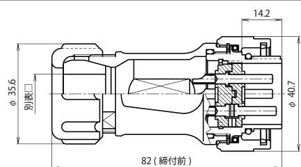
NEW-28 ■ -PM □
