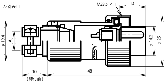
NWPC-16 ■ -PM □ -CH
