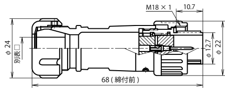
NJW-16 ■ -PM □
