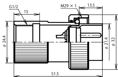
NWPC-25 ■ -GPM1/2 (注)
