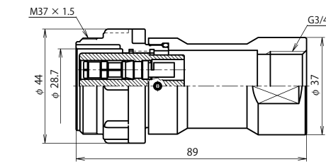
NJW-32 ■ -GAdF3/4 (注)
