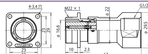
NJW-20 ■ -GAd(F)F1/2 (注)
