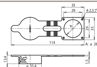
レセプタクルゴムキャップ：NRW-28-RCa・2
