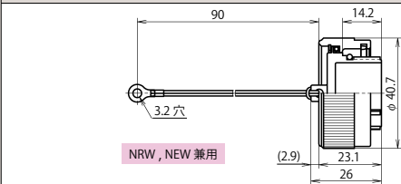
レセプタクル防水キャップ：NRW-28-RCa・1
