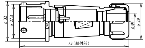
NAW-24 ■ -AdM □
