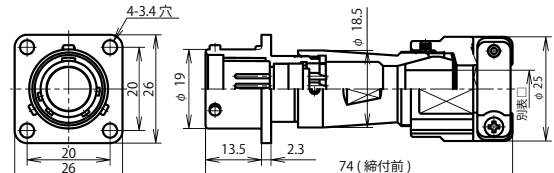
NAW-16 ■ -Ad(F)MK □
