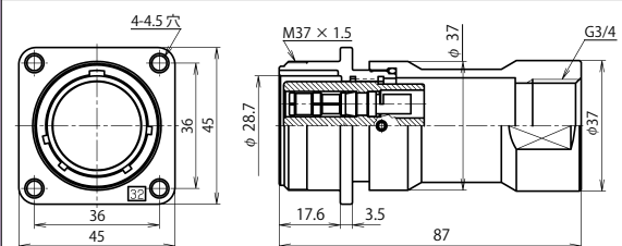
NJW-32 ■ -GAd(F)F3/4 (注)
