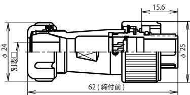
NAW-16 ■ -PF □
