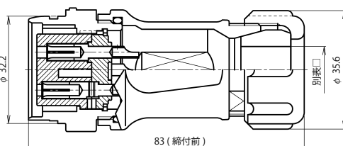
NEW-28 ■ -AdF □
