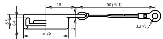
レセプタクルゴムキャップ: NRW-20-RCa
