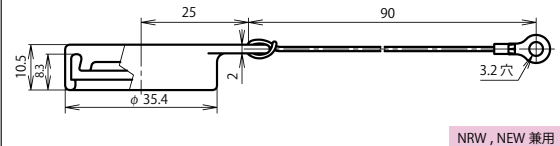
レセプタクルゴムキャップ：NRW-28-RCa
