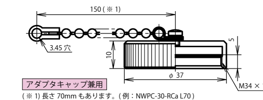
レセプタクルキャップ：NWPC-30-RCa
