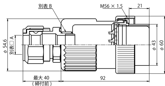
NT-50 ■ -PF □
