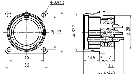
NEW-28 ■ -RM
