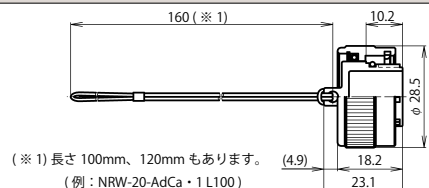
アダプタ防水キャップ：NRW-20-AdCa・1
