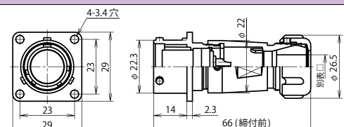
NAW-20 ■ -Ad(F)F □
