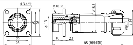
NJW-16 ■ -Ad(F)F □
