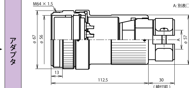
NWPC-60 ■ -AdF □
