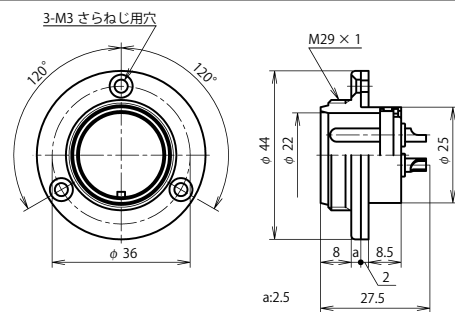
NWPC-25 ■ -R
