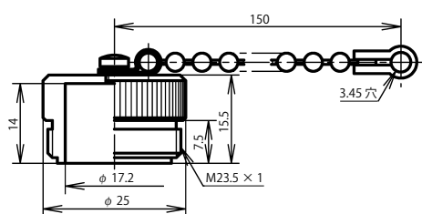
プラグキャップ：NWPC-16-PCa
