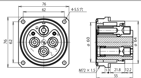
64EUMW-4RF
