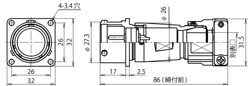
NAW-24 ■ -Ad(F)MK □
