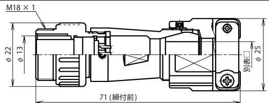
NJW-16 ■ -AdFK □
