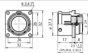
NAW-24 ■ -RM
