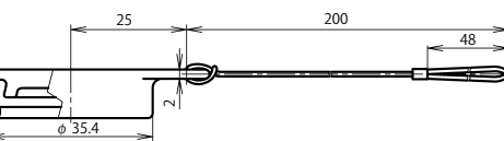
アダプタゴムキャップ：NRW-28-AdCa
