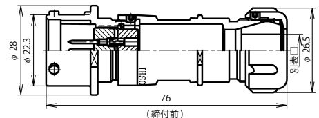
NAW-20 ■ -AdM □
