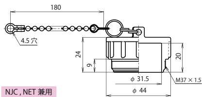
プラグキャップ：JNC-32-PCa
