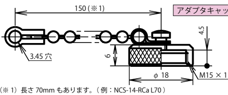
レセプタクルキャップ：NCS-14-RCa
