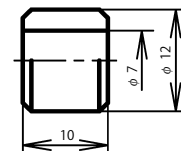
ケーブルブッシング：CBAS-12-7
