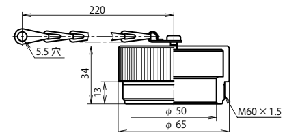
プラグキャップ：NCS-54-PCa
