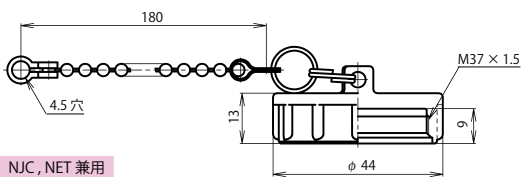
アダプタキャップ：JNC-32-AdCa
