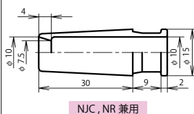
NJC, NR 兼用 ケーブルブッシング：NJC-20-CB
