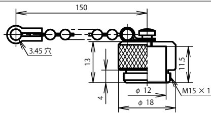
プラグキャップ：NCS-14-PCa
