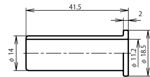
ケーブルブッシング：JJC-24-CB
