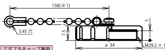
リセブタクルキャップ：NCS-30-RCa
