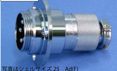
写真はシェルサイズ 25 Ad(F)
