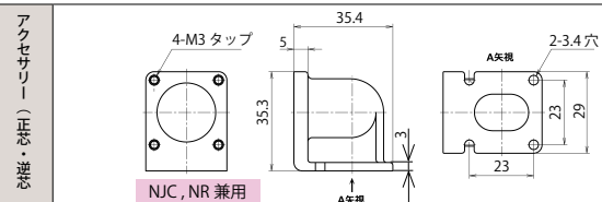
NJC, NR 兼用 NJC-20 ヨウ L ザ
