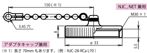
アダプタキャップ：NJC-28-RCa
