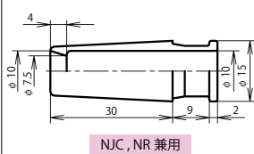
ケーブルブッシング: NJC-20-CB
