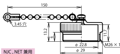
プラグキャップ：JJC-24-PCa
