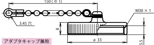
レセプタクルキャップ：NJC-28-RCa
