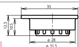
レセプタクルキャップ：NR-24-RCa・1
