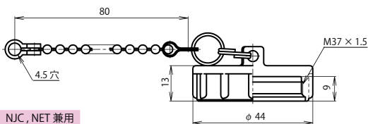
レセプタクルキャップ：JNC-32-RCa
