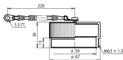
プラグキャップ：NCS-60-PCa
