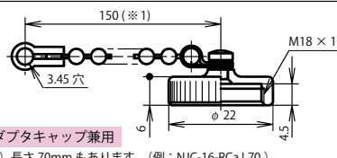
レセプタクルキャップ：NJC-16-RCa
