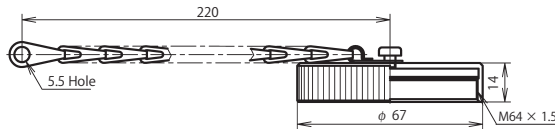
Plug cap : NWPC-60-PCa
