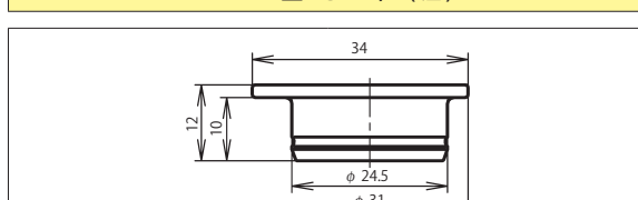
プラグキャップ：NR-24-PCa・1
