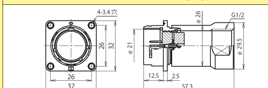
NR-24 ■ -GAd(F)M1/2 (注)
