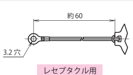
キャップヨウロープ L60
