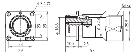
NR-20 ■ -GAd(F)F1/2 (注)
