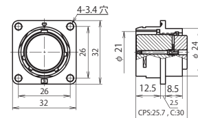
NR-24 ■ -RF
