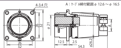
NR-24 ■ -Ad(F)F
