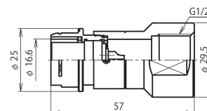
NR-20 ■ -GAdF1/2 (注)
