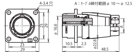
NR-20 ■ -Ad(F)F
