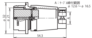
NR-24 ■ -AdF
