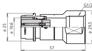
NR-20 ■ -GAdF1/2 (注)
