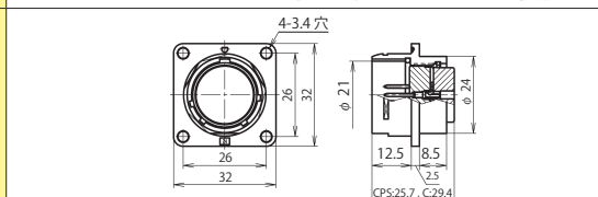
NR-24 ■ -RM
