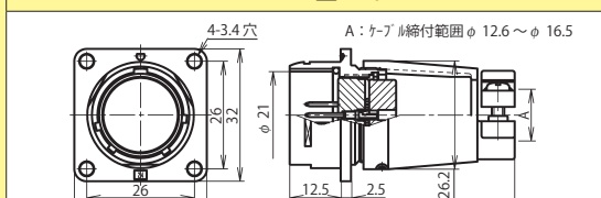
NR-24 ■ -Ad(F)M
