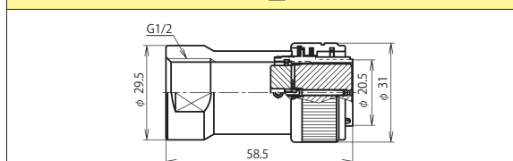
NR-24 ■ -GPF1/2 (注)
