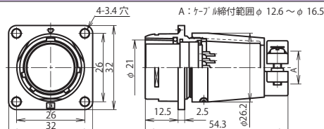
NR-24 ■ -Ad(F)F
