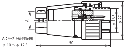
NR-20 ■ -PM
