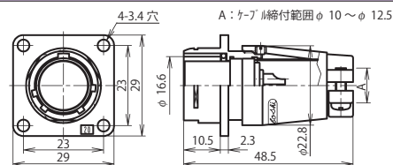
NR-20 ■ -Ad(F)F
