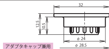
レセプタクルキャップ：NR-20-RCa・1
