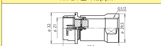
NR-24 ■ -GAdM1/2 (注)
