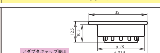
レセプタクルキャップ：NR-24-RCa・1
