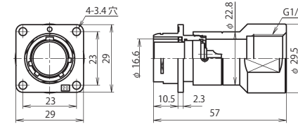
NR-20 ■ -GAd(F)F1/2 (注)
