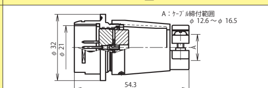
NR-24 ■ -AdM
