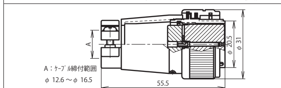
NR-24 ■ -PF
