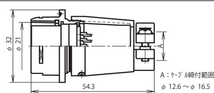
NR-24 ■ -AdF
