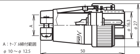
NR-20 ■ -PM
