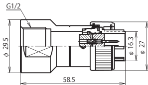
NR-20 ■ -GPM1/2 (注)
