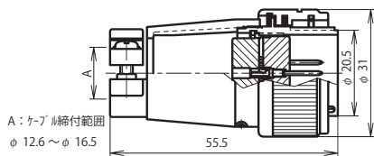
NR-24 ■ -PM
