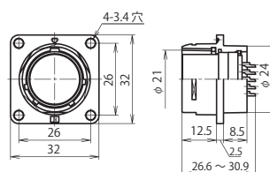
NR-24 ■ -RF
