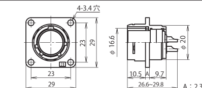
NR-20 ■ -RF
