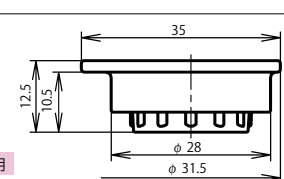
アダプタキャップ兼用 レセプタクルキャップ：NR-24-RCa・1
