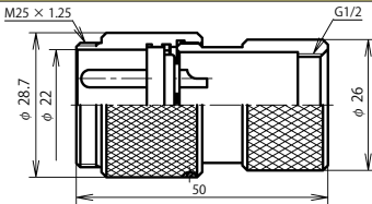
NCS-25 ■ -GAd1/2 (注)
