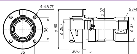
BWC-32 ■ -GAd(F)F3/4 (注)
