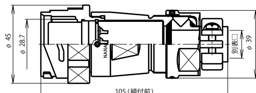
BWC-32 ■ -AdF □
