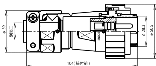
BWC-32 ■ -PM □
