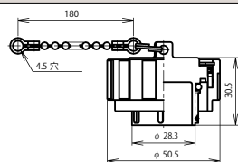
アダプタキャップ：BWC-32-AdCa
