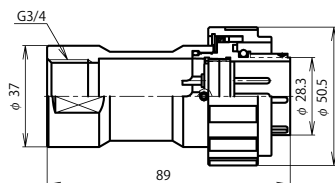
BWC-32 ■ -GPM3/4 (注)
