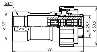
BWC-32 ■ -GPF3/4 (注)
