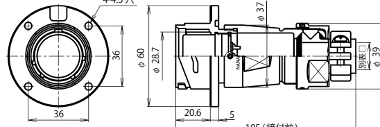
BWC-32 ■ -Ad(F)F □
