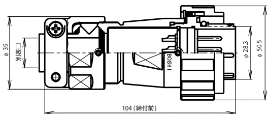
BWC-32 ■ -PM □
