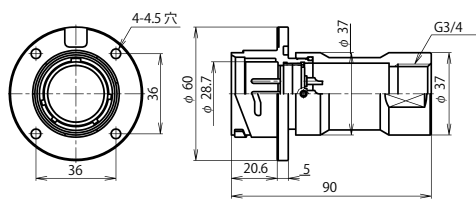
BWC-32 ■ -GAd(F)M3/4 (注)
