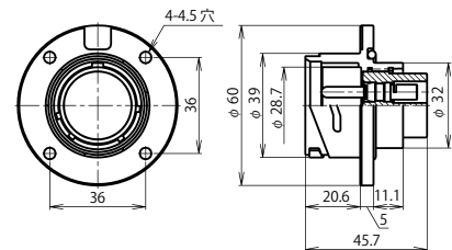
BWC-32 ■ -RM
