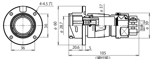
BWC-32 ■ -Ad(F)M □
