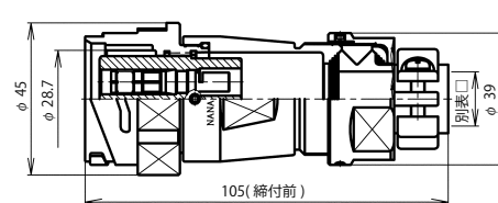
BWC-32 ■ -AdF □
