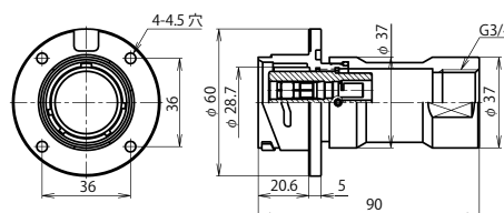
BWC-32 ■ -GAd(F)F3/4 (注)
