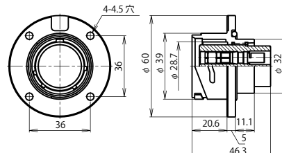
BWC-32 ■ -RF
