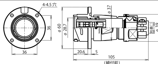
BWC-32 ■ -Ad(F)F □
