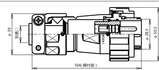
BWC-32 ■ -PF □
