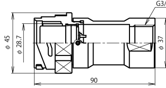
BWC-32 ■ -GAdF3/4 (注)
