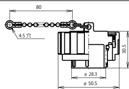
レセプタクルキャップ：BWC-32-RCa
