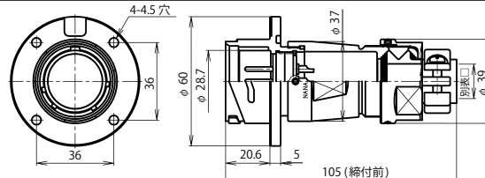
BWC-32 ■ -Ad(F)M □
