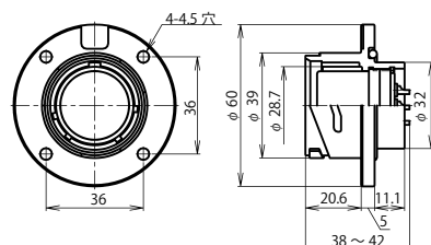
BWC-32 ■ -RF
