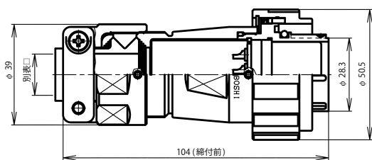
BWC-32 ■ -PF □
