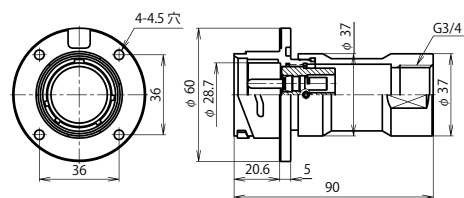
BWC-32 ■ -GAd(F)M3/4 (注)
