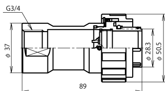
BWC-32 ■ -GPF3/4 (注)
