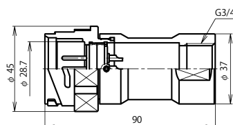
BWC-32 ■ -GAdM3/4 (注)
