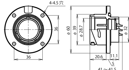
BWC-32 ■ -RM
