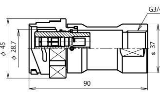
BWC-32 ■ -GAdF3/4 (注)
