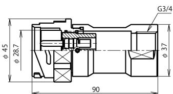
BWC-32 ■ -GAdM3/4 (注)
